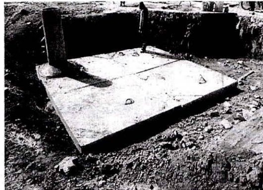
Interligação da rede existente com nova rede.
