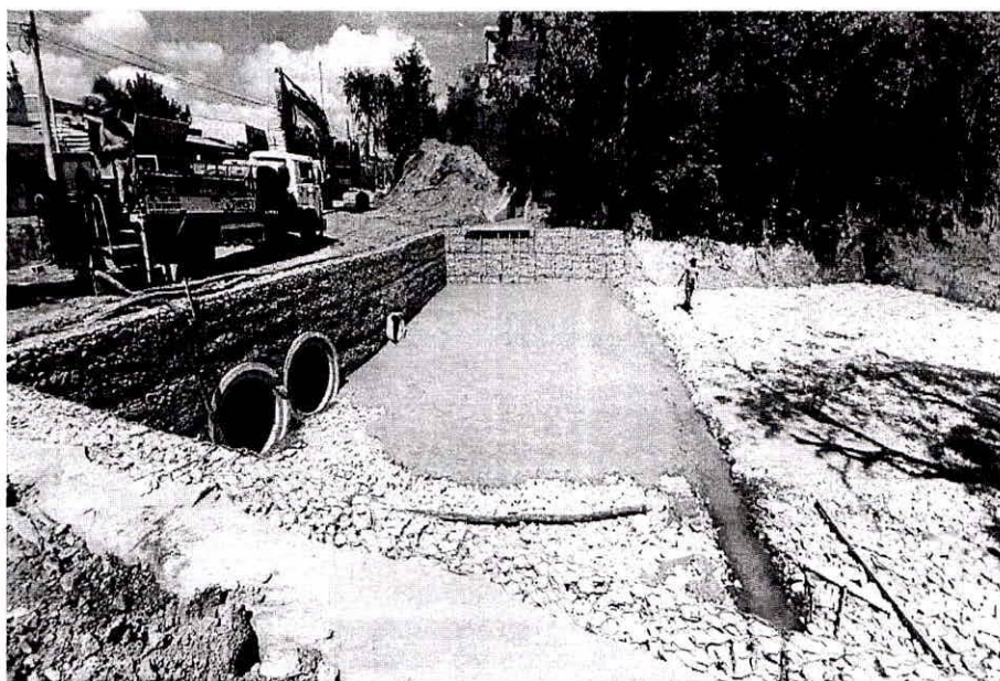
Tanque de captação
